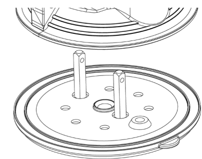
CAOUTCHOUC REMPLAÇABLE AUSTAUSCHBARES GUMMI
