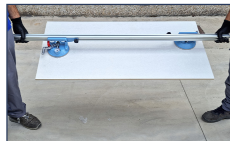
Possibilité de travailler même sans poignées surélevées. Es ist möglich, auch ohne erhöhte Griffe zu arbeiten.
