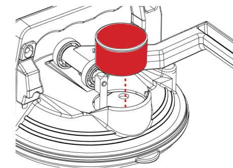
VACUOMÈTRE REMPLAÇABLE AUSTAUSCHBARES VAKUUMMETER
