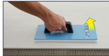
Fliesen-Fugbrett 16x33 cm zum korrekten Ausstoßen der Luft unter der Fliese.
